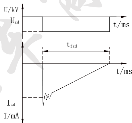
图5 齐纳放电波形示例
